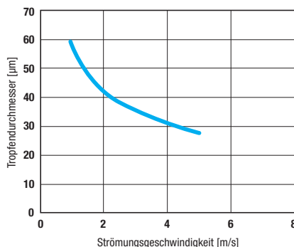
Grenztropfengröße DV 270
