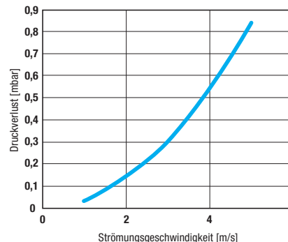
Druckverlust DV 270
